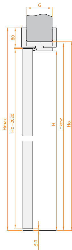
PRZEKRÓJ PIONOWY
